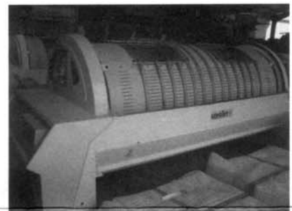
Pressoir mécanique VASLIN
